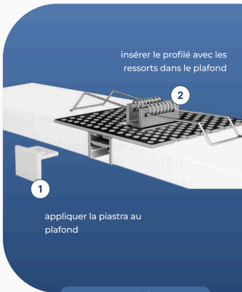
piastra avec ressort CL-RS16/01
